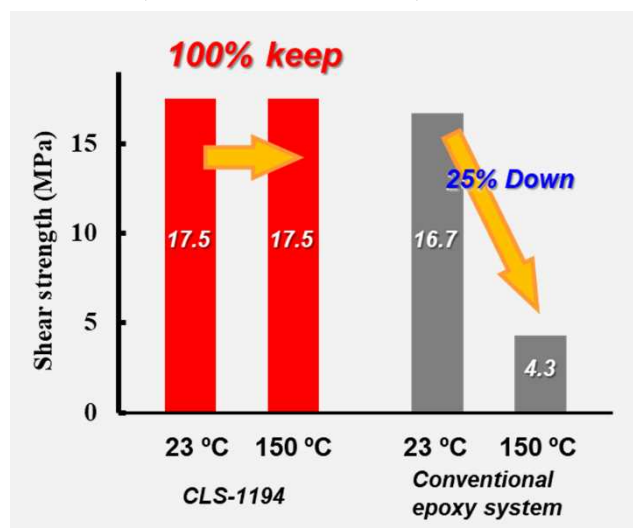
Fe/Fe 剪断接着試験 (180 °C × 1 hr)
