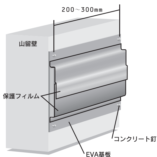
施工方法
